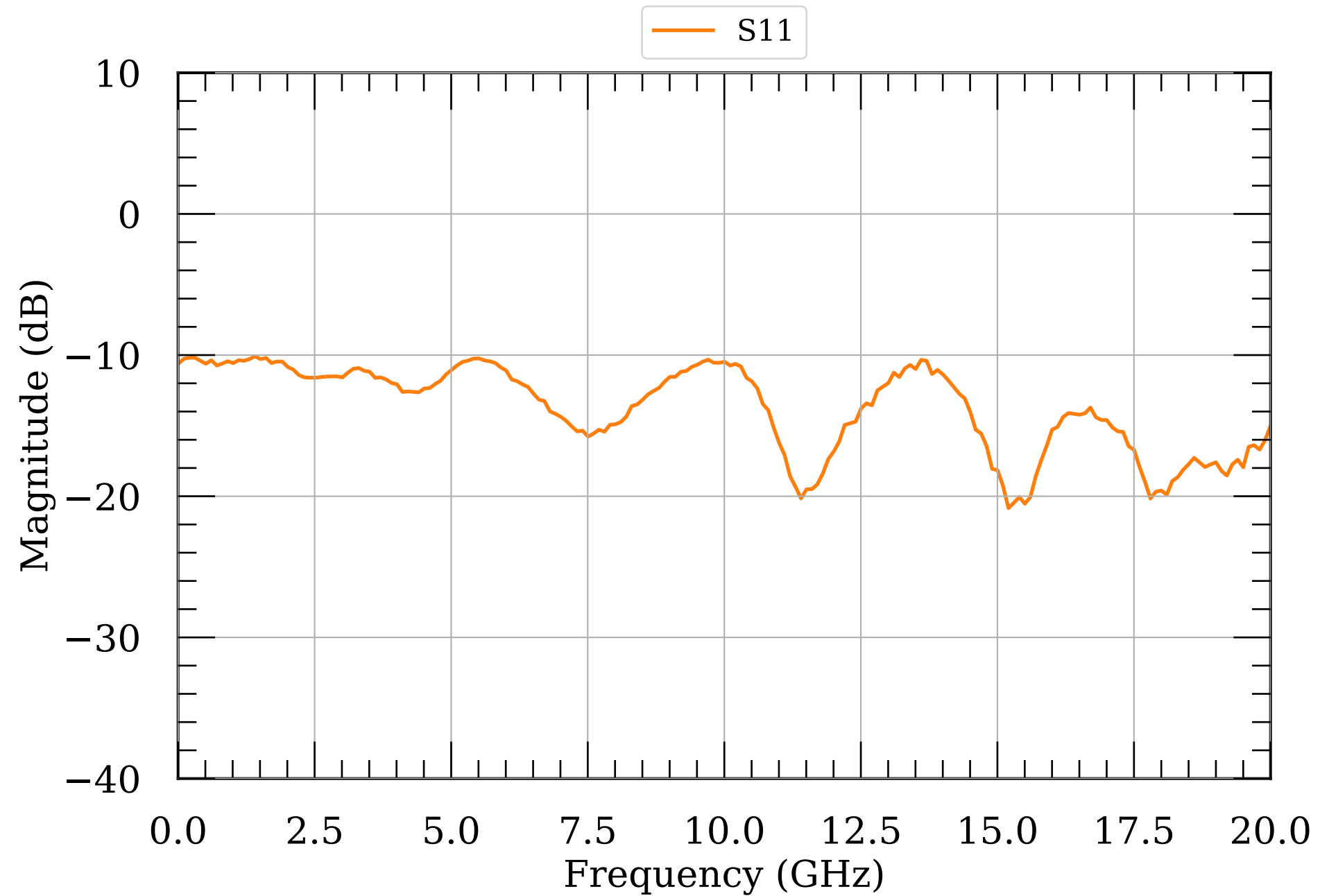
LNA S-params module084v2
